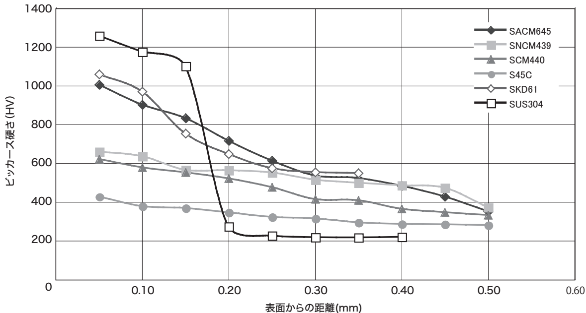
鋼種別硬度推移曲線(2段窒化48時間処理)
