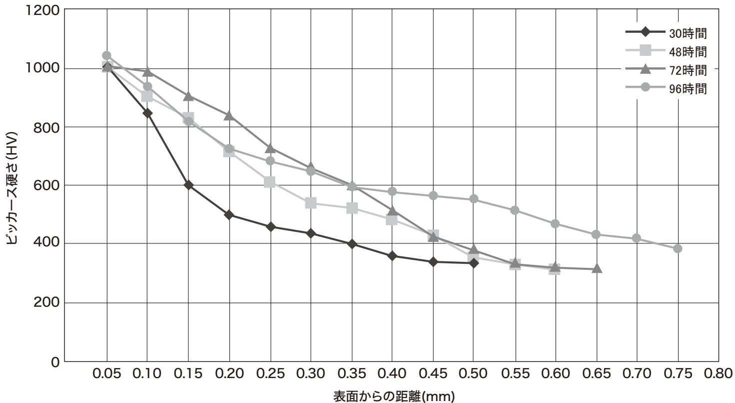
処理時間の差異による硬度推移曲線 (材質SACM645)
